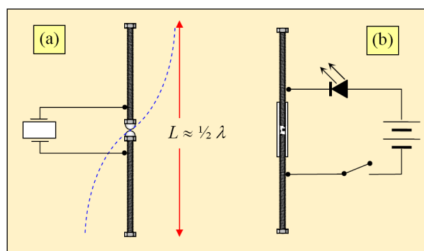
Figura 3. (a) Emisor. Está formado por un encendedor piezoeléctrico y un dipolo. (b) Detector. Consta de un cohesor, interruptor, dos pilas de 1,5 V y LED.
