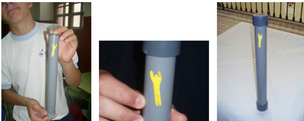
Figura 4. (Izq.) Un alumno muestra una imagen del escalador subiendo. (Centro) Detalle del muñequito, que está hecho con la portada de un cuaderno. (Der.) Otra imagen del escalador magnético, en la que se aprecia claramente los tapones especiales para tubos de PVC.
