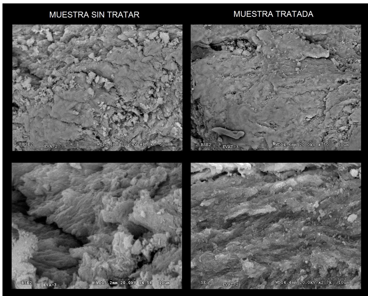
Figura 4. Microfotografía electrónica de barrido. SEM
