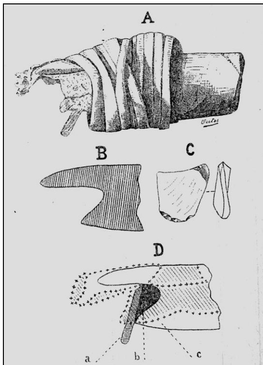
Figura 5. Dibujo de raspador Selk' Nam, tomado de Outes, 1906. A. conjunto. B. corte del mango. C. raspador de vidrio. D. modo de fijación
