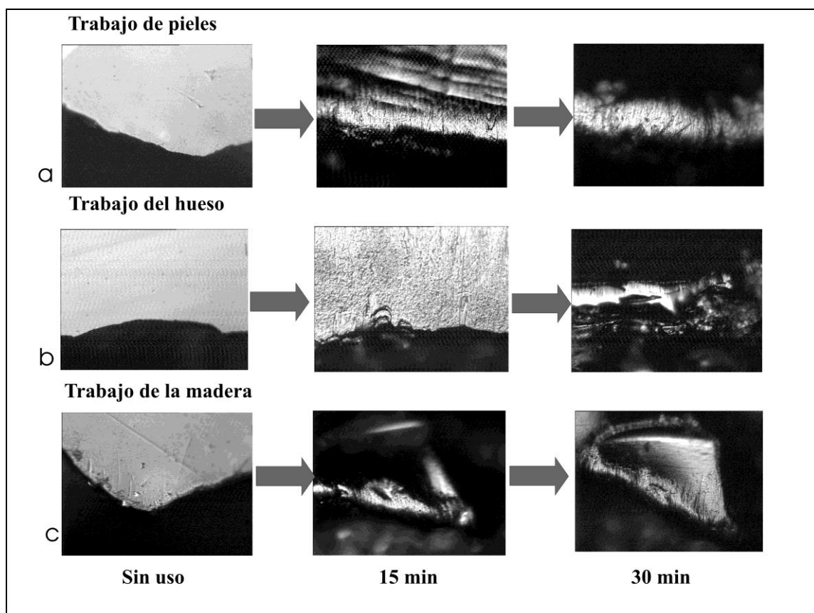
Figura 12. Modificación de la microtopografía durante el proceso de uso. Fotomicrografías de filos de tres raspadores de vidrio tomadas a diferentes intervalos, 200 X
